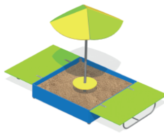
С крышкой и зонтом Артикул: ИСУ-05.01.02 Размеры ДхШхВ: 1,5x1,5x2
