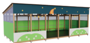
«Небо» брус Артикул: МАФ-02.03.02 Размеры ДхШхВ: 9х4,75х3,185 Полезная площадь: 38,1 м2
