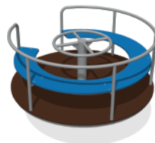
Со сплошным сиденьем Артикул: ИСУ-08.12 Размеры ДхШхВ: 1,67х1,67х0,8
