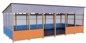
«Бюджетная 3» брус Артикул: МАФ-02.02.05.06 Размеры ДхШхВ: 9х4,75х3,185 Полезная площадь: 38,1 м2
