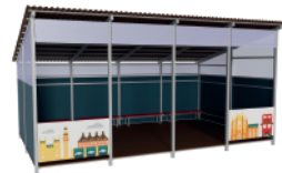
«Англия» металл Артикул: МАФ-02.01.23.03 Размеры ДхШхВ: 6х4,2х3,2 Полезная площадь: 21 м2
