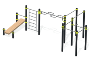
«Воркаут 6» Артикул: СОУ-02.20 Размеры ДхШхВ: 5,7x2,9x2,6
