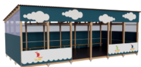
«Бриз» брус Артикул: МАФ-02.03.01 Размеры ДхШхВ: 9х4,75х3,185 Полезная площадь: 38,1 м2
