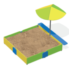
«Полдень» Артикул: ИСУ-05.07 Размеры ДхШхВ: 2,6x2x1,95 (песочница 2x2x0,35)
