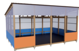
«Бюджетная 1» брус Артикул: МАФ-02.02.05.04 Размеры ДхШхВ: 6х4,75х3,185 Полезная площадь: 25,55 м2
