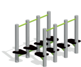
«Шагоход» Артикул: СОУ-01.11 Размеры ДхШхВ: 1,65х0,8х1
