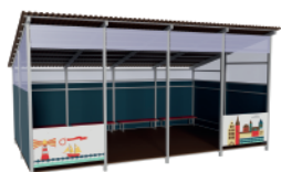
«Нидерланды» металл Артикул: МАФ-02.01.23.04 Размеры ДхШхВ: 6х4,2х3,2 Полезная площадь: 21 м2
