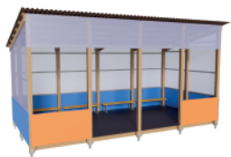
«Бюджетная 2» брус Артикул: МАФ-02.02.05.05 Размеры ДхШхВ: 6х3,5х3,2 Полезная площадь: 17,25 м2
