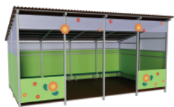
«Гербера» металл Артикул: МАФ-02.01.22.02 Размеры ДхШхВ: 6х4,2х3,2 Полезная площадь: 21 м2
