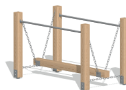
Качающееся бревно Артикул: COY-01.47 Размеры ДхШхВ: 1,5х0,9х1,1
