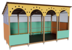
«Арлекин» Артикул: МАФ-02.02.04 Размеры ДхШхВ: 6х3,5х3,2 Полезная площадь: 17,25 м2
