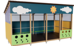
«Весна» брус Артикул: МАФ-02.02.00 Размеры ДхШхВ: 6х3,5х3,2 Полезная площадь: 17,25 м2
