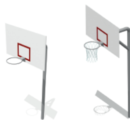
«Щит баскетбольный» детский, взрослый Артикул: СОУ-01.1 Артикул: СОУ-01.20 Размеры ДхШхВ: 1,2х0,8х1,8 Размеры ДхШхВ: 1,8х1,8х3,95
