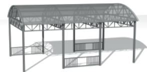
Навес для тренажерной площадки с секциями ограждений Артикул: МАФ-03.01 Размеры ДхШхВ: 5,56х8,5х3,8
