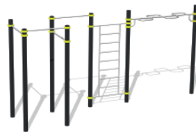
«Воркаут 1» Артикул: СОУ-02.15 Размеры ДхШхВ: 5,6x1,5x2,55
