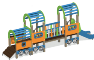
«Локомотив с вагончиком» Артикул: ИСУ-11.13.02 Размеры ДхШхВ: 5,75х1,45х2,4 высота ската 0,8м
